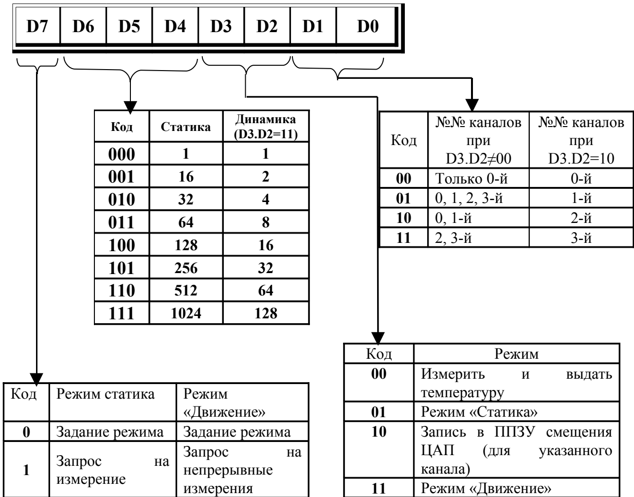
Рис.3 Управляющее слово для СИМ-А04.10
