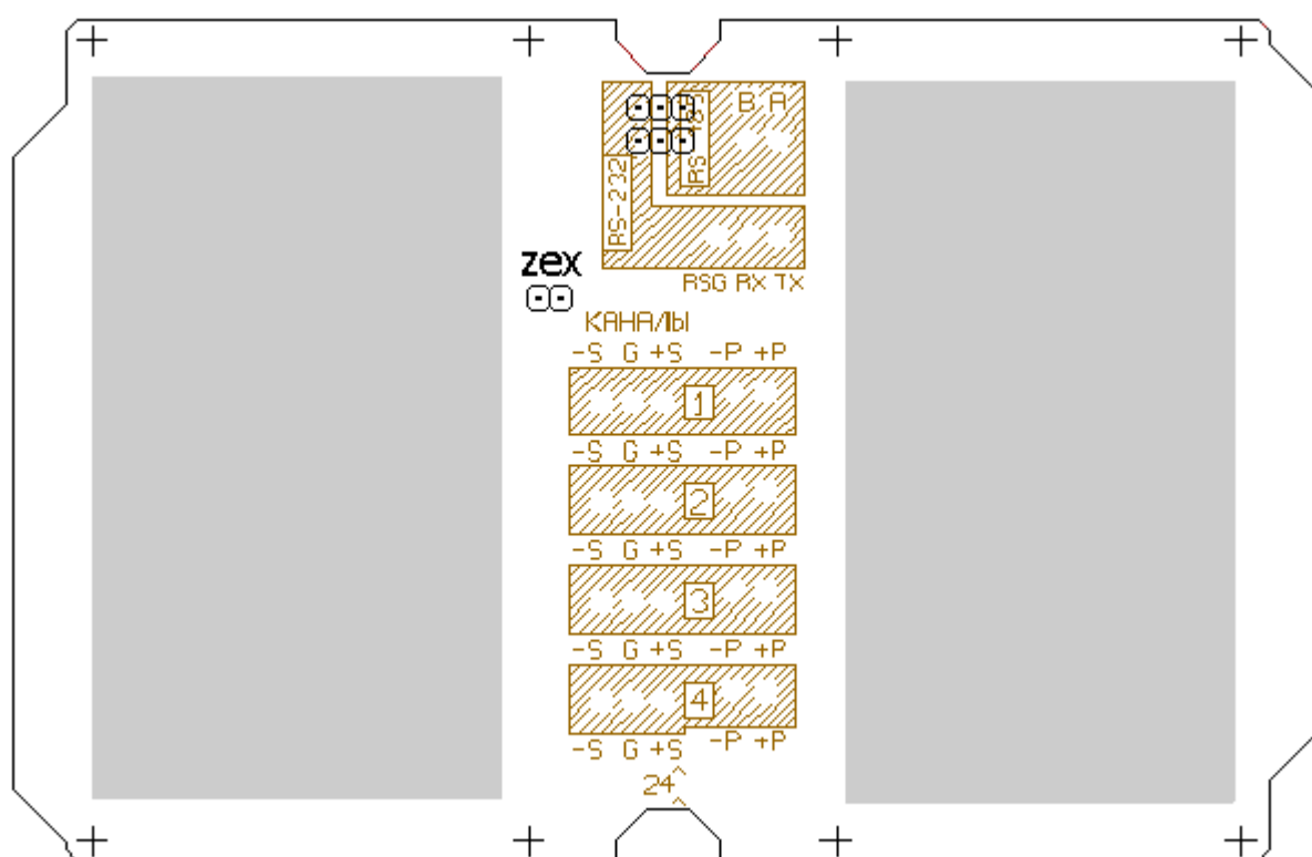
Рис.3. Размещение клемм подключения и перемычек на плате СИМ-А04.10
